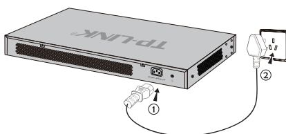
图3-3 电源线连接示意图
