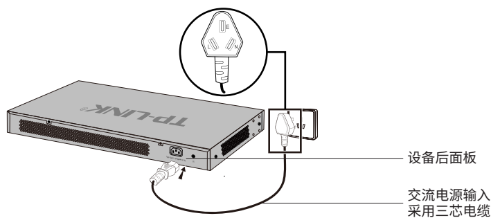
图2-5 PE线连接示意图
