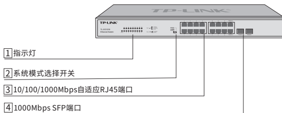
图1-1 前面板示意图
